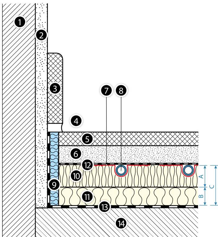
Obr. 31. Podlahová otopná plocha se systémovou deskou KAN-therm TBS a doplňkovou izolací a hydroizolační vrstvou na desce položené na terénu
