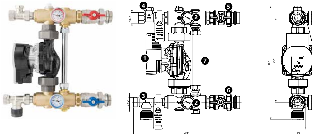
Obr. 54. Konstrukce čerpadlového systému KAN-therm.
