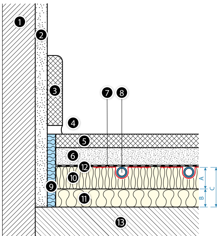
Obr. 30. Podlahové topné těleso se systémovou deskou KAN-therm TBS a doplňkovou izolací na stropě nad vnitřní místností a na stropě, který sousedícím se vnějším vzduchem.
