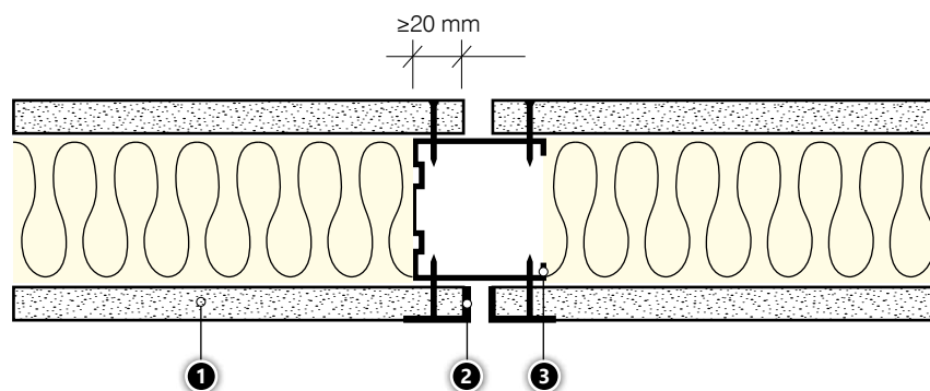
Obr. 42. Otevřená mezera.
