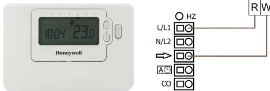
Obr. 67. Schéma svorek a připojení 7denního regulátoru 24 V - 230 V k elektrické sběrnici Basic+.
