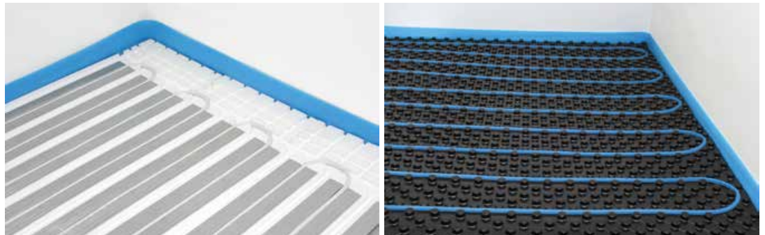
Obr. 13. Příklady okrajové izolace u podlahového vytápění KAN-therm.
