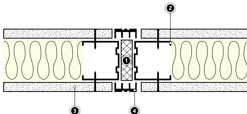
Obr. 43. Dilatační spára.
