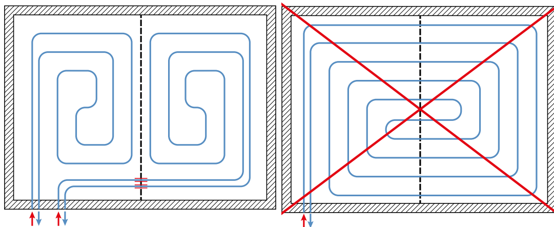
Obr. 19. Správné a chybné rozdělení otopné plochy dilatační spárou
