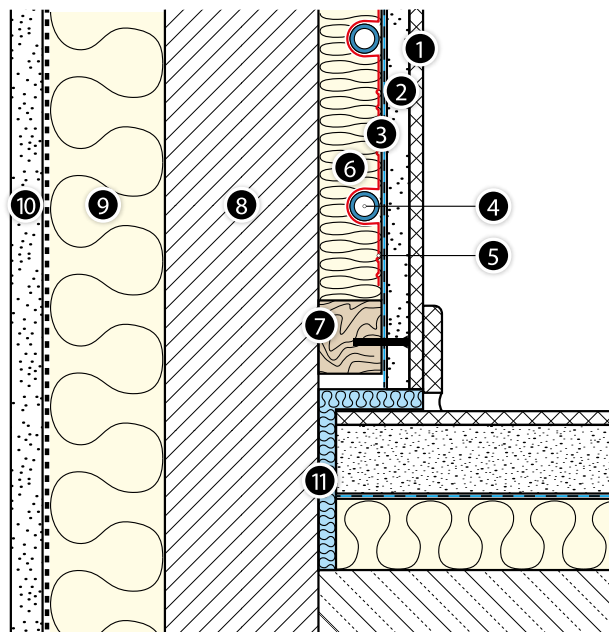
Obr. 36. Konstrukce stěnového vytápění KAN-therm TBS.
