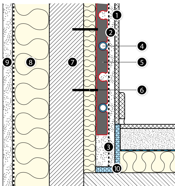
Obr. 35. Konstrukce instalace stěnového vytápění/chlazení KAN-therm Rail
