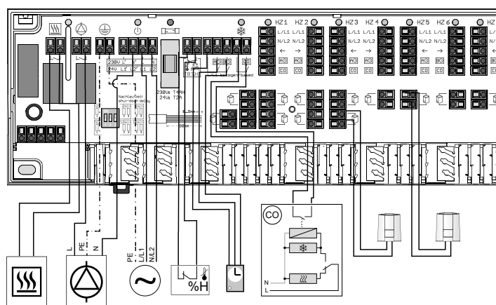
Obr. 72. Konfigurace elektrické sběrnice Basic+ 230 V nebo 24 V s čerpadlovým modulem, modulem kotle a periferními zařízeními.
