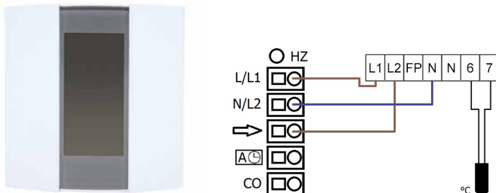
Obr. 68. Schéma svorek a připojení týdenního termostatu TH232-AF.
