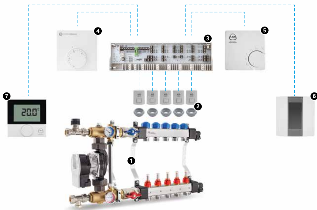
Obr. 60. Příklad lokálního nastavení vedení a automatiky KAN-therm v plošném vytápění.
