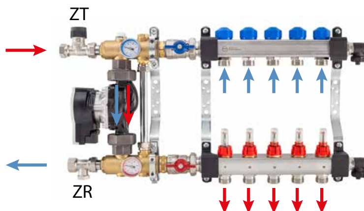
Obr. 57. Rozdělovač se směšovací jednotkou USFP – směry průtoků.
