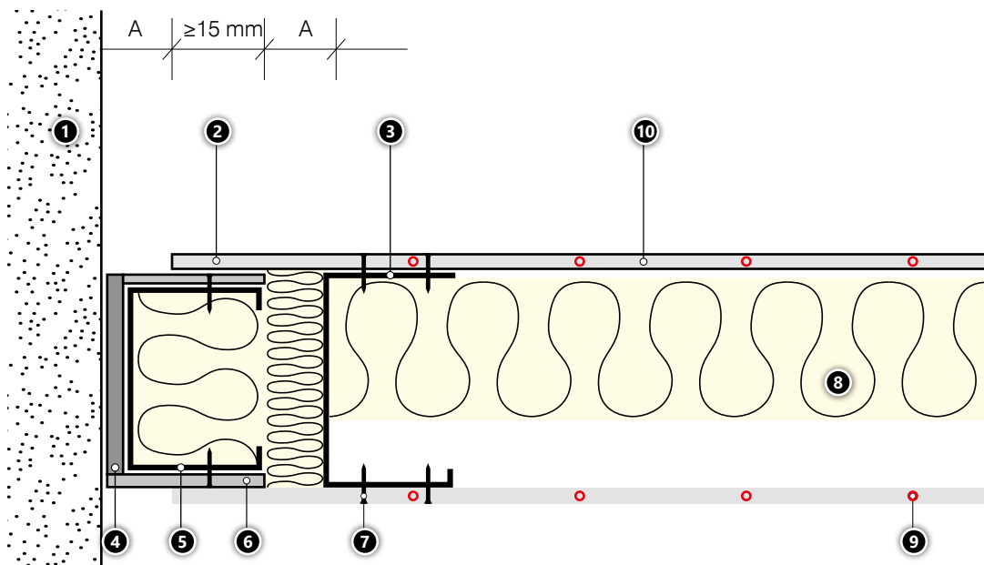
Obr. 41. Posuvný spoj se stěnou.
