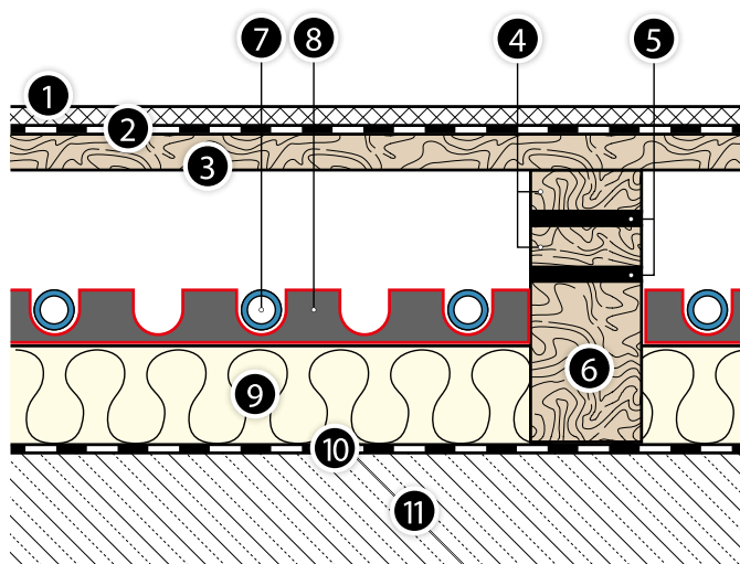
Obr. 33. Řez plošně pružnou sportovní podlahou se soustavou podlahového topení realizovanou z prvků systému KAN-therm Rail
