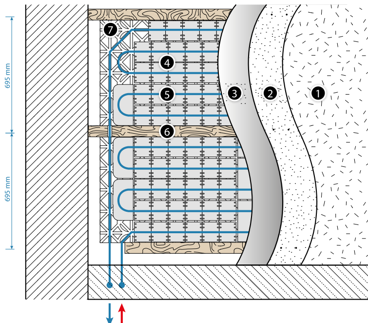
Obr. 37. Průřez instalace stěnového vytápění KAN-therm TBS.
