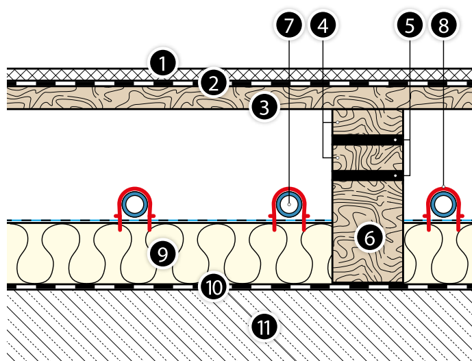
Obr. 32. Řez plošně pružnou sportovní podlahou se soustavou podlahového topení realizovanou z prvků systému KAN-therm Tacker.
