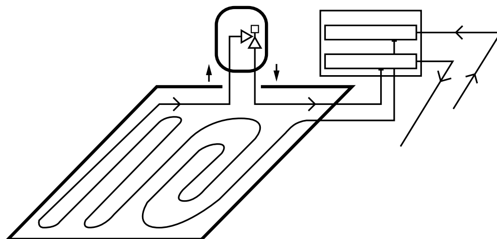
Obr. 77. Schéma fungování – skupina umístěná na vratném potrubí
