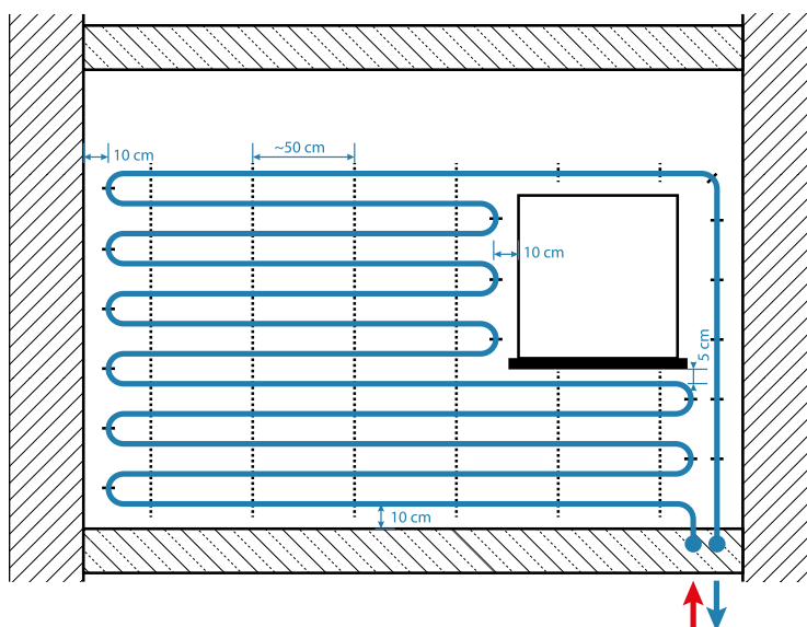
Obr. 34. Montážní vzdálenosti u stěnového vytápění.
