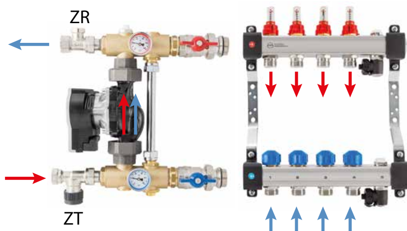
Obr. 58. Čerpadlová skupina se stálými hodnotami s rozdělovačem UFST – směry průtoků.
