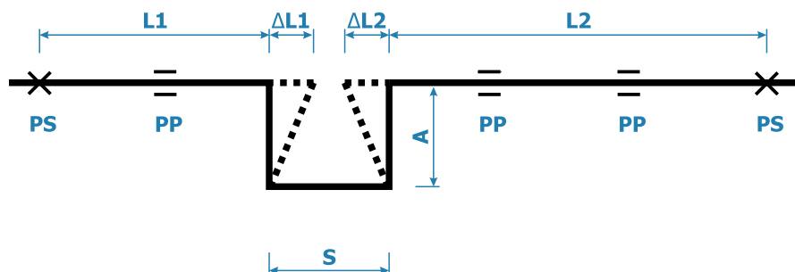
Kompensátor tvaru U pro ocelové trubky
