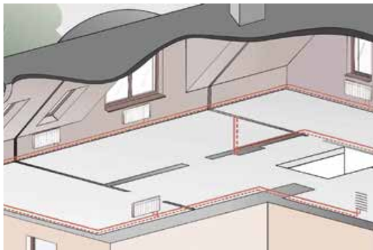
Dvoutrubkový okruhový rozvod otopné soustavy
